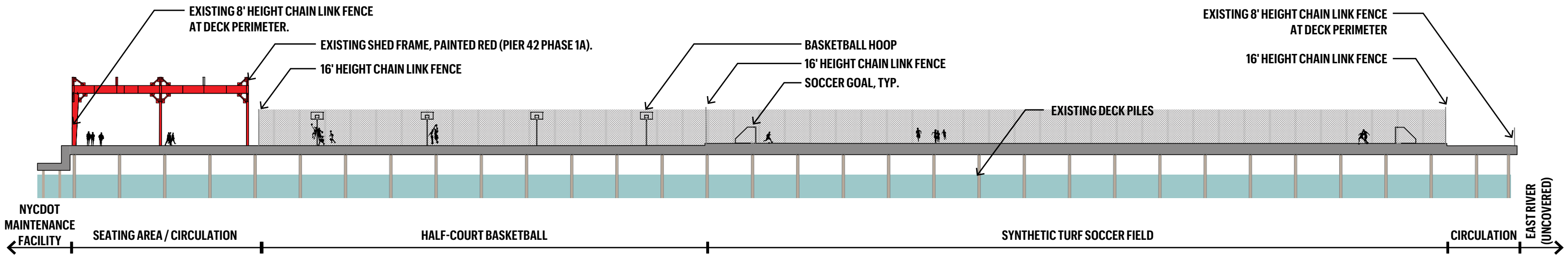
SECTION A-A'
