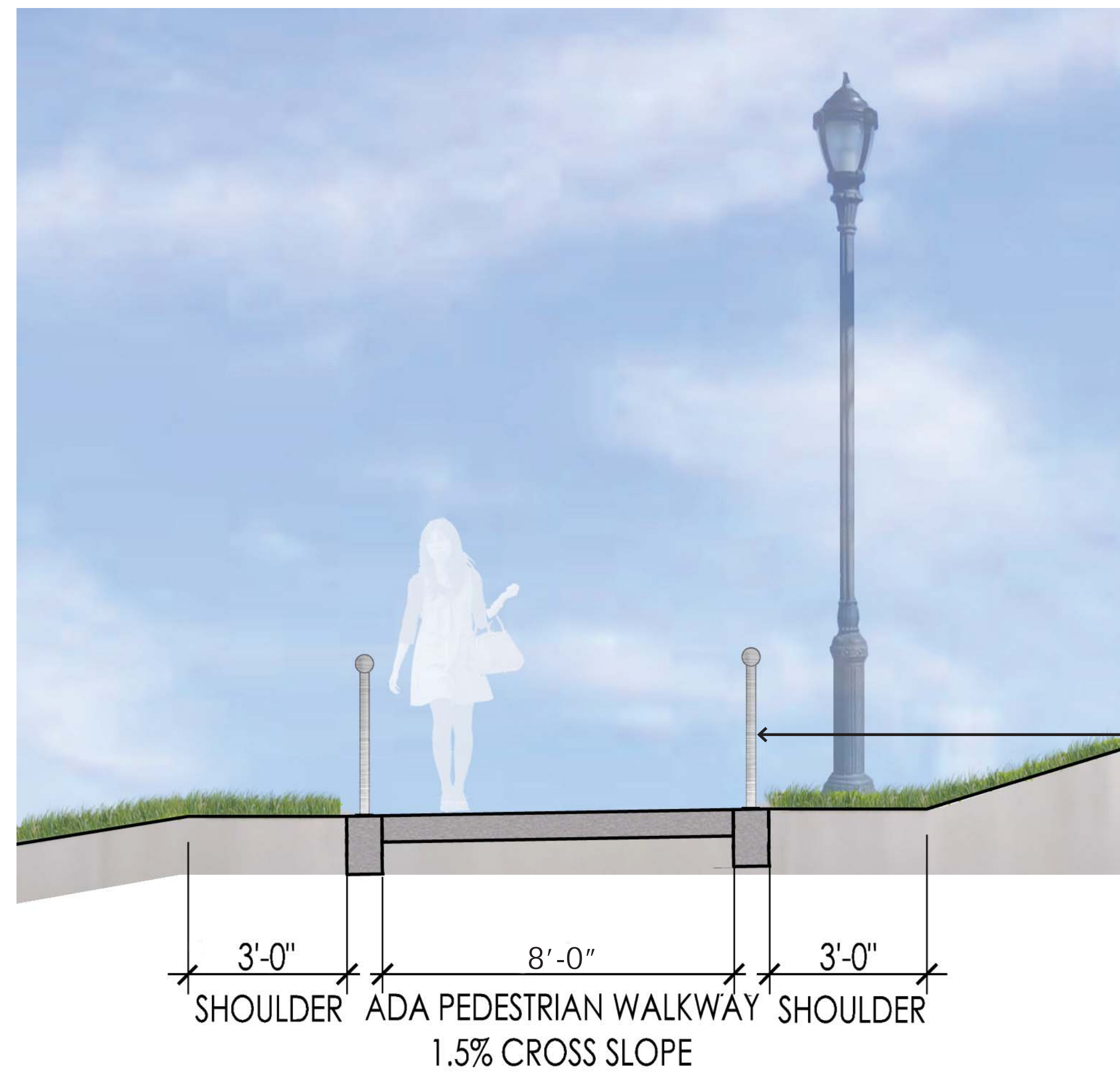
ADA PATH SECTION N.T.S
