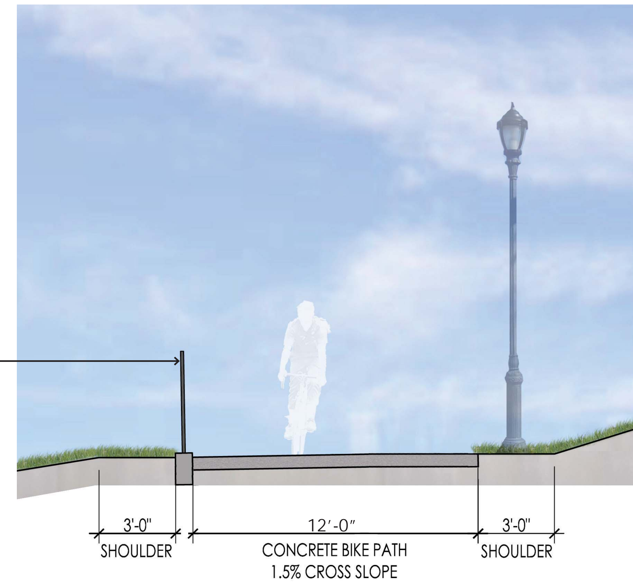
BIKE PATH SECTION N.T.S
