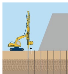
灯芯排水管安装
