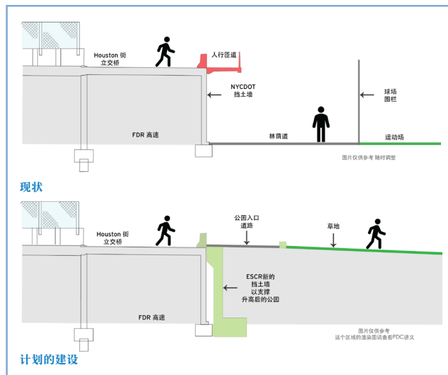
东Houston街立交桥挡土墙的现状和计划建设的示意图
