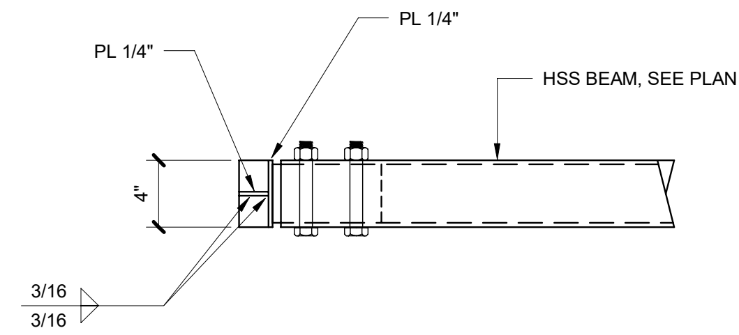
SECTION - 2A
