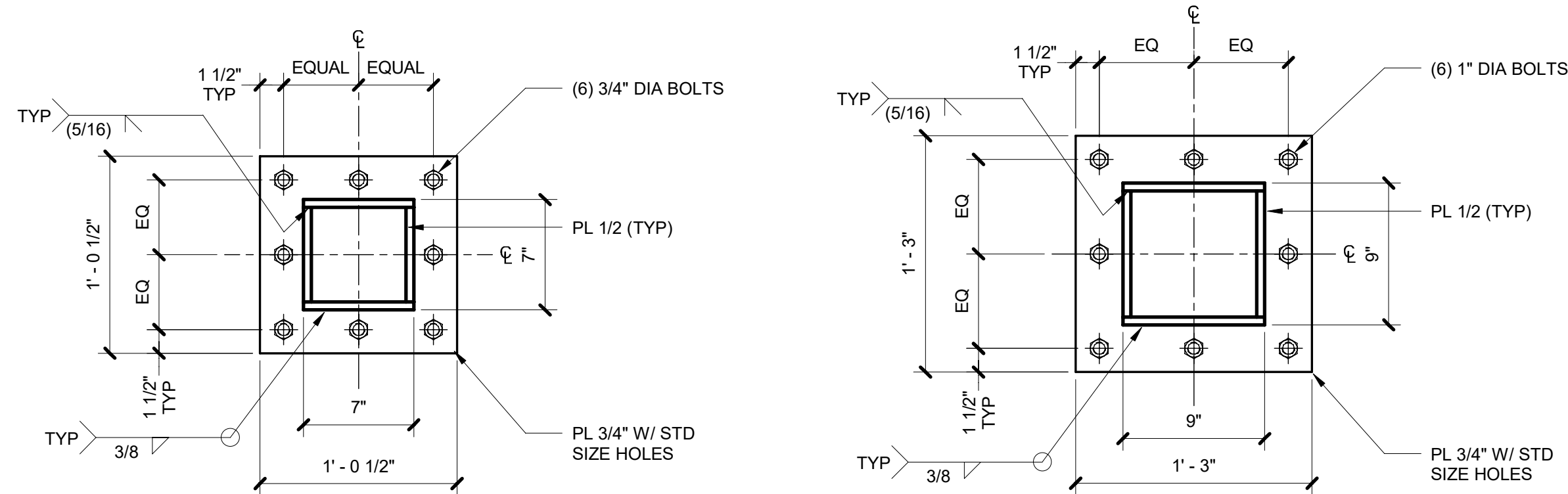
SECTION - 1E
