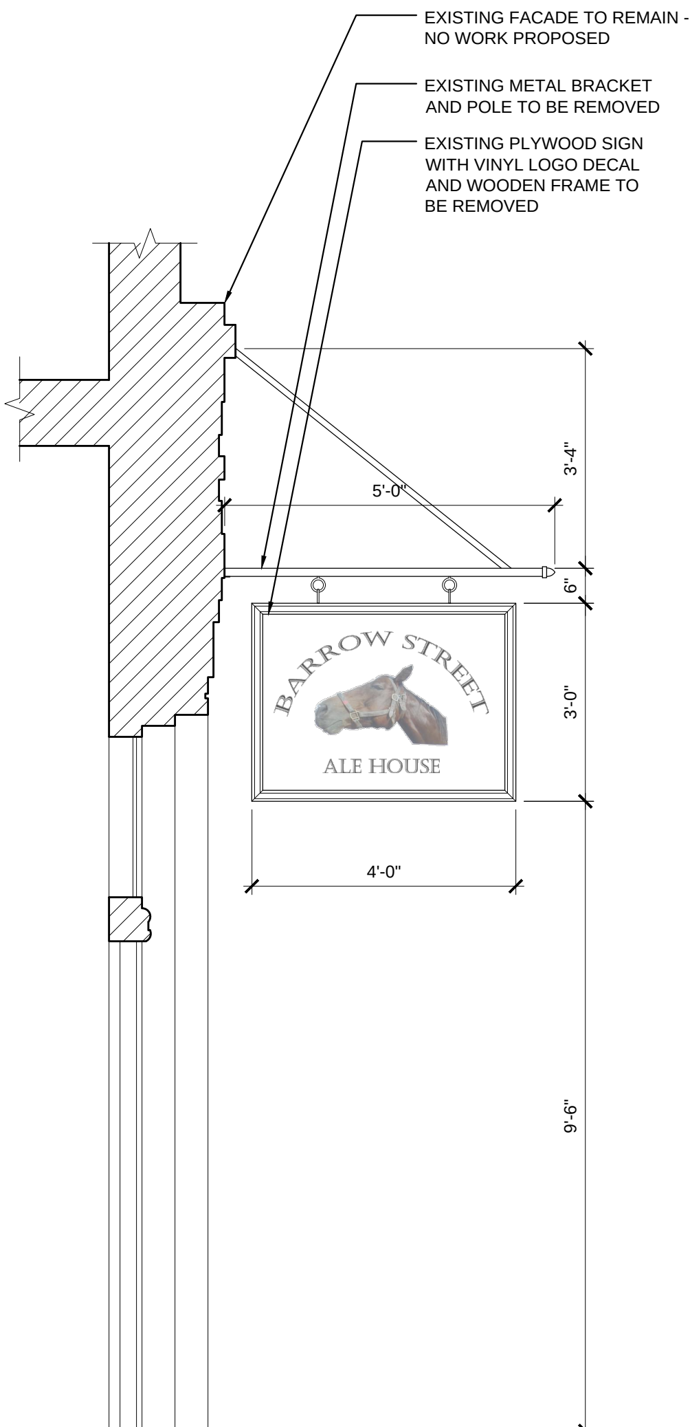
2 EXISTING SECTION A-101 SCALE: 1/2"=1'-0"
